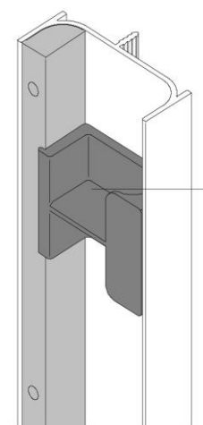
Montážní pomůcka
