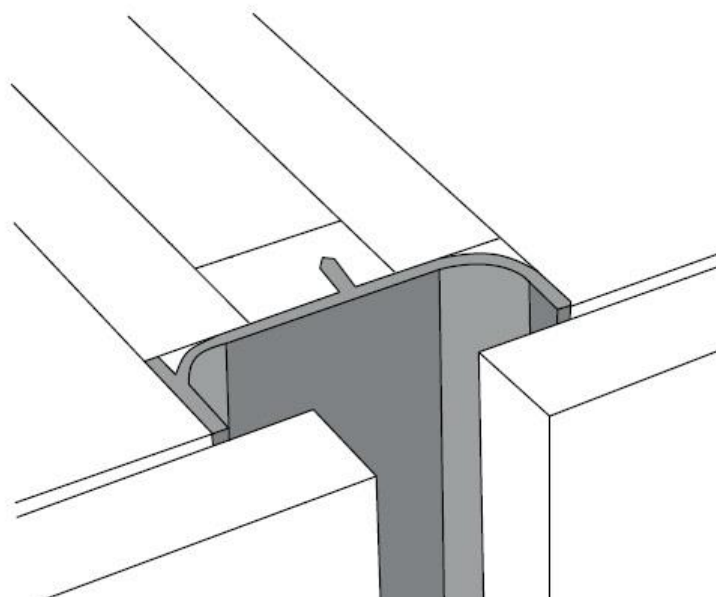
UKÁZKA POUŽITÍ VERTIKÁLNÍHO PROFILU „ J „
